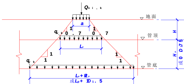
图 C.0.3 考虑结构整体作用时 车辆荷载的竖向压力传递分布
