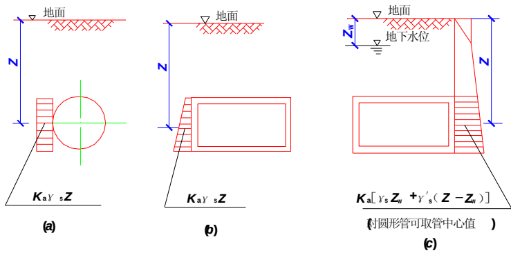
图 3.2.3 作用在管道上的侧向土压力 (a) 圆形管道 (无地下水); (b) 矩形管道 (无地下水); (c) 管道埋设在地下水位以下
